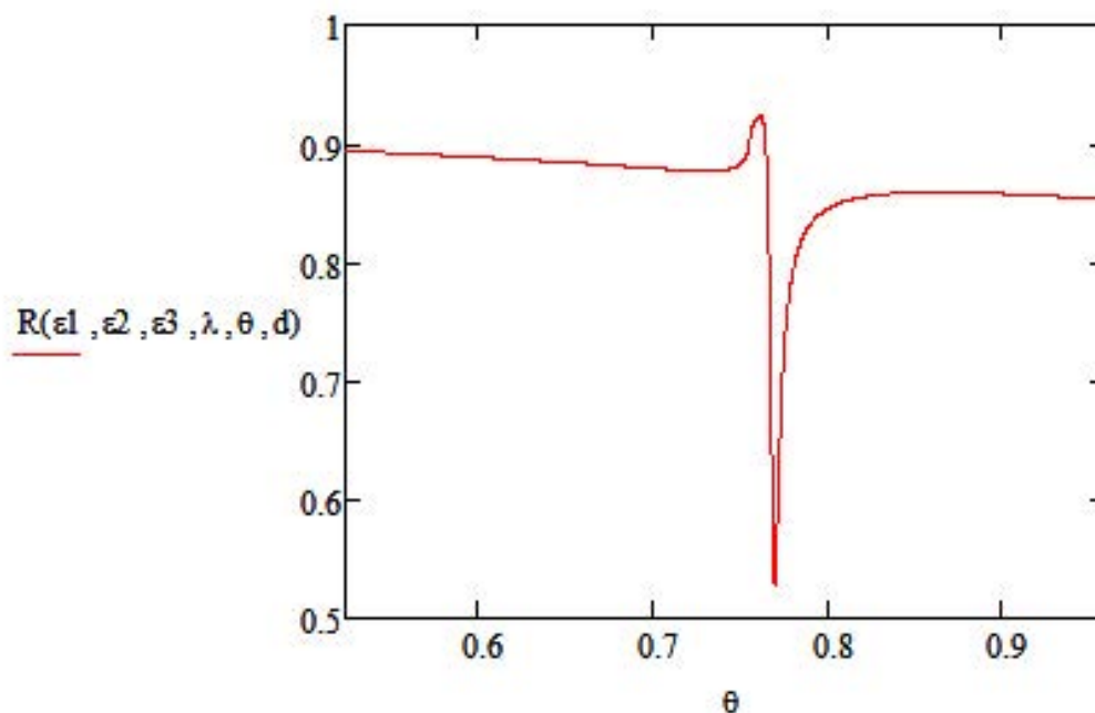
Рис.3. Зависимость коэффициента отражения 3-х-слойной структуры с гетерогенным слоем (GaAs-Ag) от угла падения излучения с длиной волны 0.8.мкм.
