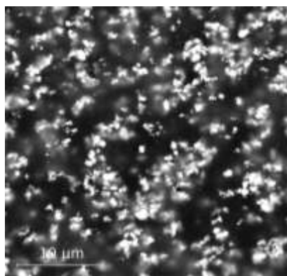
Рис. 3. СЭМ изображения поверхности композита: а), она же после сегментации по методу Оцу б).
