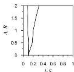
Рис. 4. Границы клюва синхронизации, измеренные в ходе обработки временных рядов колебаний напряжения на выходе ГЗОС, возбуждаемого внешним сигналом с частотой, изменяющейся по нелинейному закону для амплитуд внешнего воздействия 0.5 В, 1 В, 1.5 В и 2.0 В.
