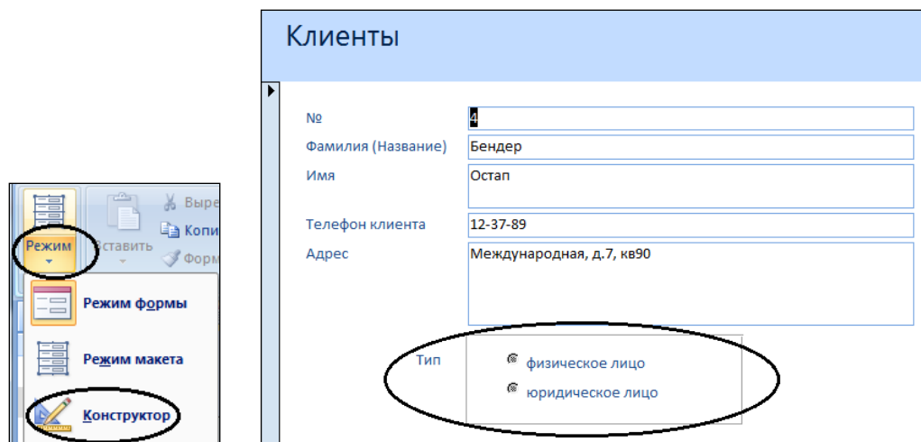
Рис.1.53. Режим формы
