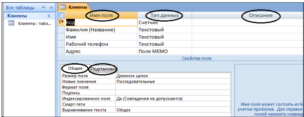
Рис.1.19. Окно Конструктора
