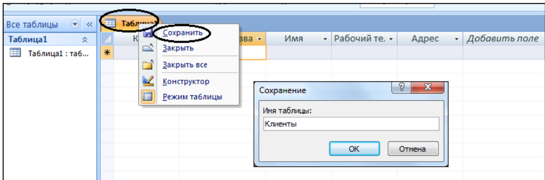
Рис.1.10. Сохранение таблицы
