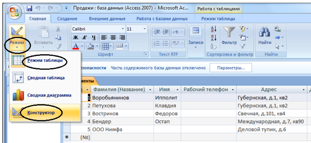
Рис.1.18. Кнопка Конструктор
