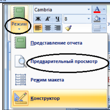
Рис.1.63. Конструктор отчета
