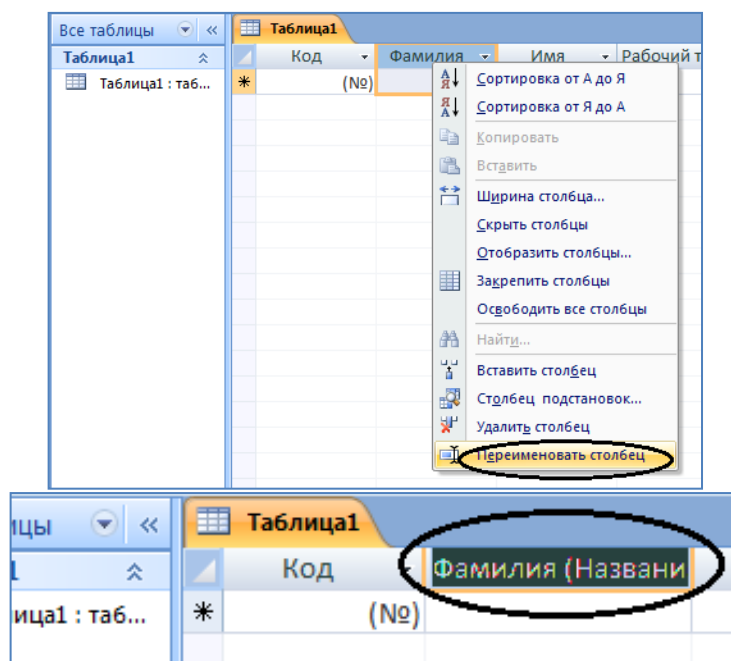
Рис.1.9. Переименование поля
