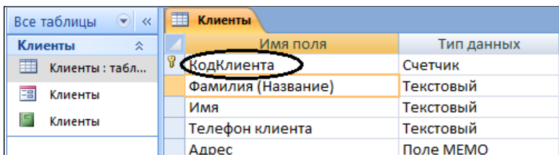
Рис.1.65. Переименование поля
