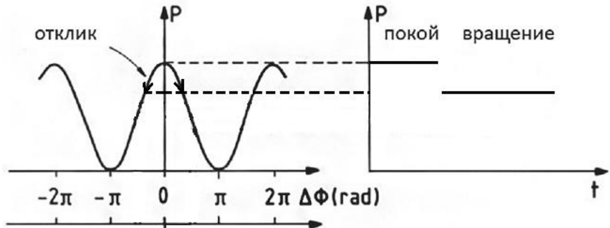
Рисунок 1.2 - Передаточная характеристика интерферометра Саньяка
