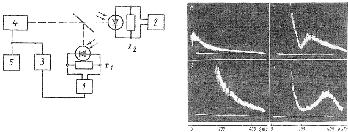
Рисунок 2.1 - Блок-схема системы шумоподавления по методу с обратной связью по току накачки и спектрограммы шума выходного сигнала измерительного канала интерферометра: а - спектр дробового шума фотоприемника; б - спектр сигнала без шумоподавления; в, г - спектры сигнала с небольшой и максимальной обратной связью, из статьи [65]
