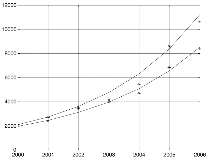
Рис. 1 Исходные данные по расходной и доходной части бюджета (звездочки) и результаты решения для математической модели (непрерывные линии). Цветом выделены: зеленым — расходная часть бюджета, синим — доходная. По оси абсцисс отложено время в годах, по оси ординат — части бюджета в миллиардах рублей.
